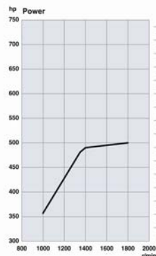
DC16 18 560 Euro 5
