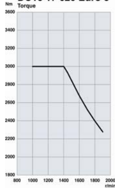
DC16 17 620 Euro 5
